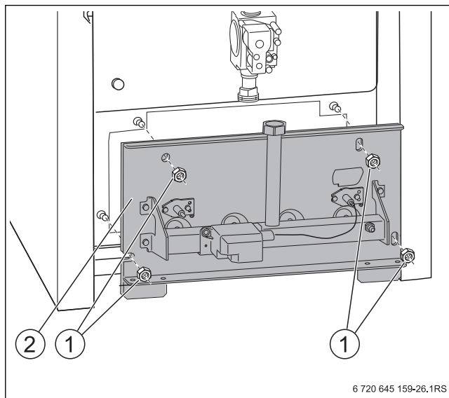
Рис. 45 Снятие крепежных гаек
