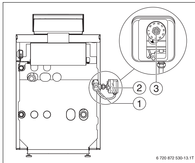
Рис. 50 Установка реле контроля давления газа
