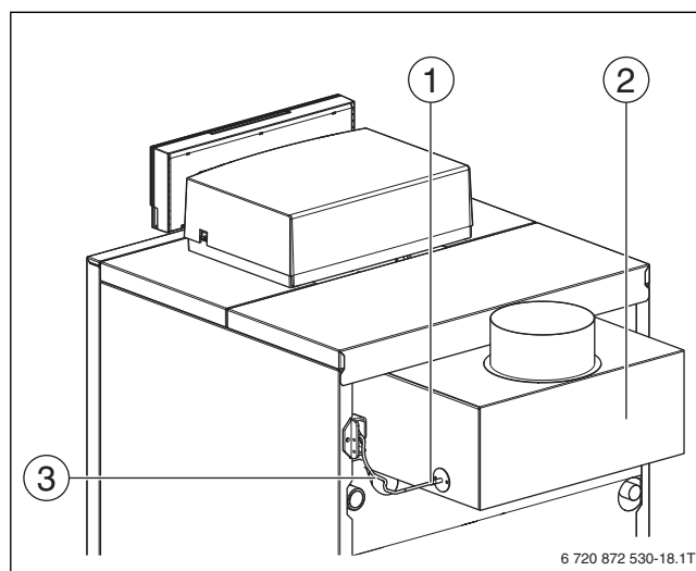
Рис. 13 Датчик контроля дымовых газов
