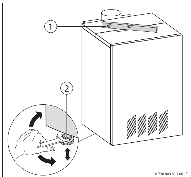
Рис. 9 Выравнивание котла
