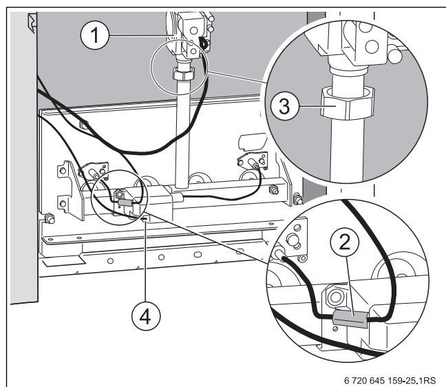
Рис. 44 Демонтаж горелки
