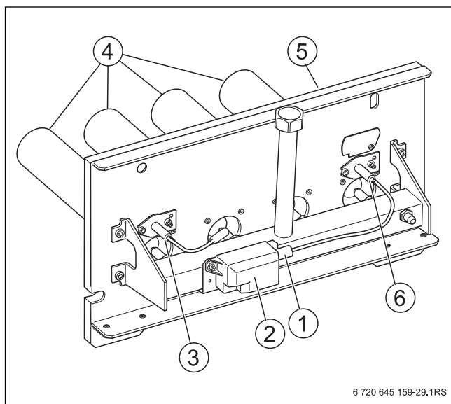
Рис. 48 Чистка горелки
