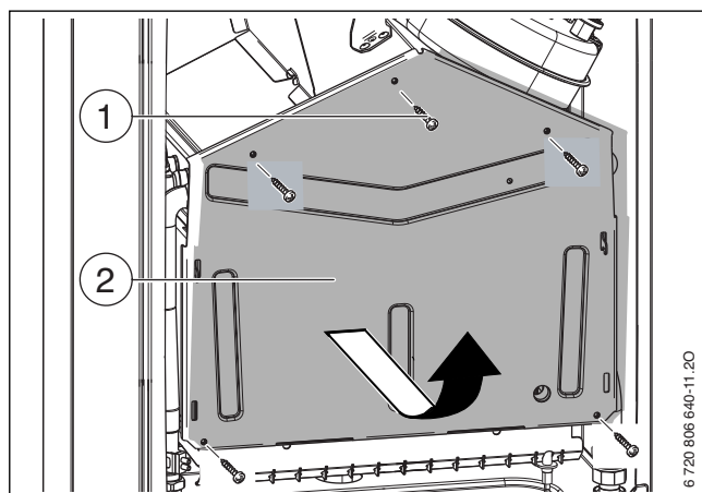
Рис. 39 Открытие горелки
