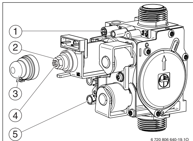
Рис. 32 Газовая арматура
