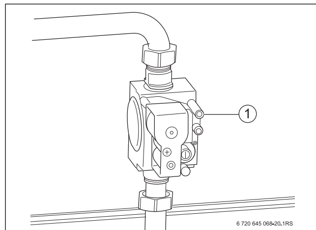
Рис. 30 Измерение подаваемого давления газа
