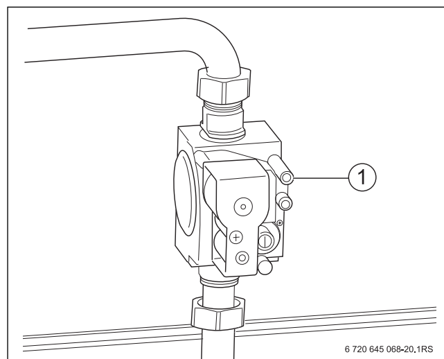
Рис. 26 Удаление воздуха из газопровода
