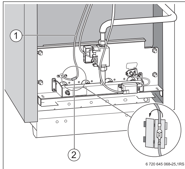
Рис. 32 Удаление защиты от касания
