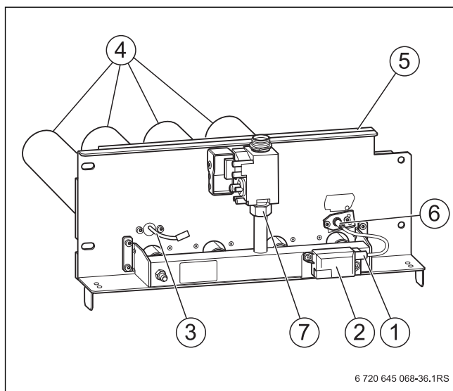
Рис. 46 Чистка горелки
